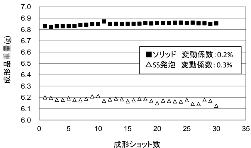
図 2 非発泡成形(ソリッド)とショートショット発泡(「RIC-FOAM」SS 発泡、軽量化率:10wt%)成形の連続成形での成形品重量変動 樹脂:タルク強化ポリプロピレン樹脂(タルク 20wt%) 金型:40mm×60mm、t=2mm、平板金型
