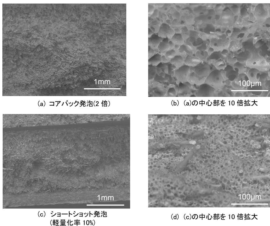
図 3 PPS(ガラスフィラー30wt%)樹脂での発泡成形品(コアバック発泡、ショートショット発泡)の断面写真(発泡ガス:窒素(6MPa)) (破断面を表面走査電子顕微鏡で観察)
