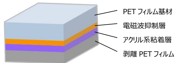
透明導電塗料を採用した薄膜透明電磁波抑制粘着フィルム
